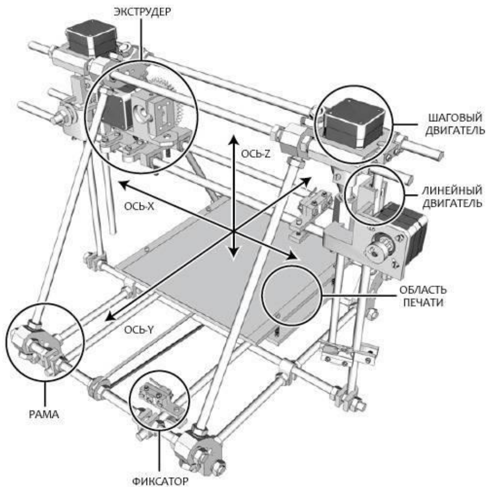
Схема 3D-принтера.
